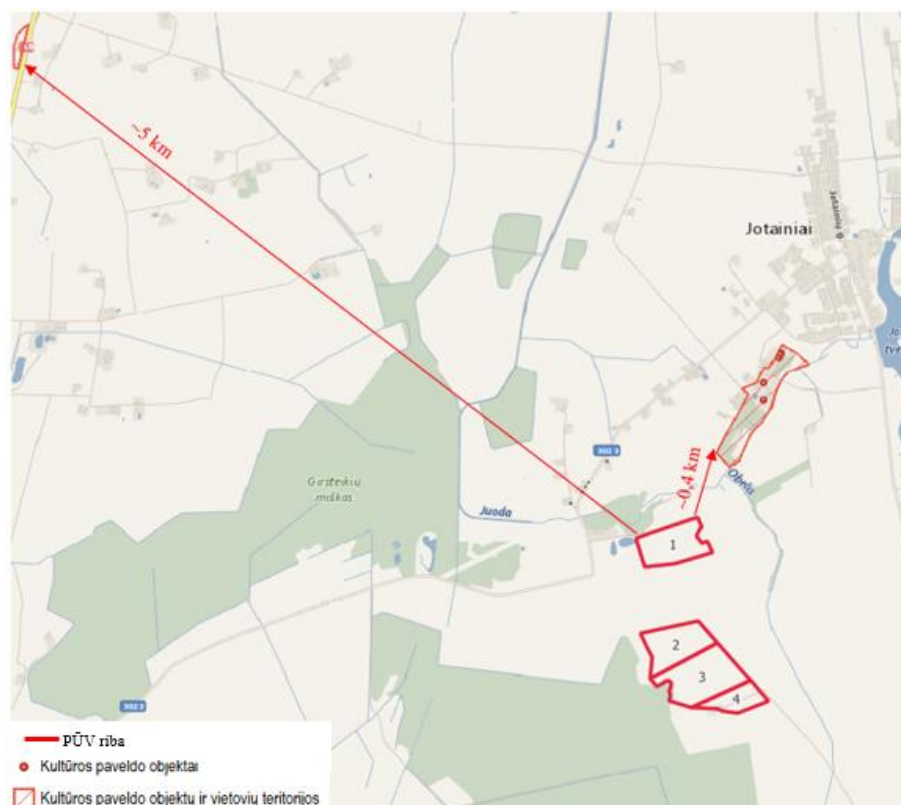
2.49 pav. Ištrauka iš kultūros vertybių registro žemėlapis (Šaltinis: kvr.kpd.lt/#/static-heritage-search )
