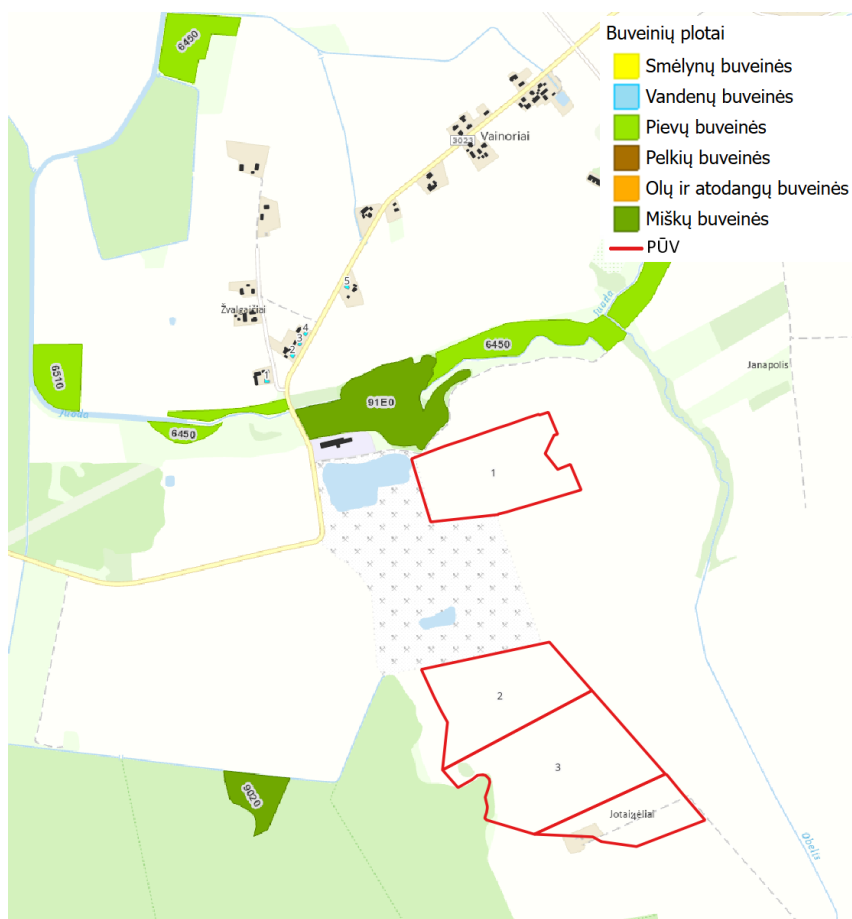
2.19 pav. Ištrauka iš Europos bendrijos svarbos natūralių buveinių inventorizacijos žemėlapiu (Šaltinis: https://www.geoportal.lt/ )
