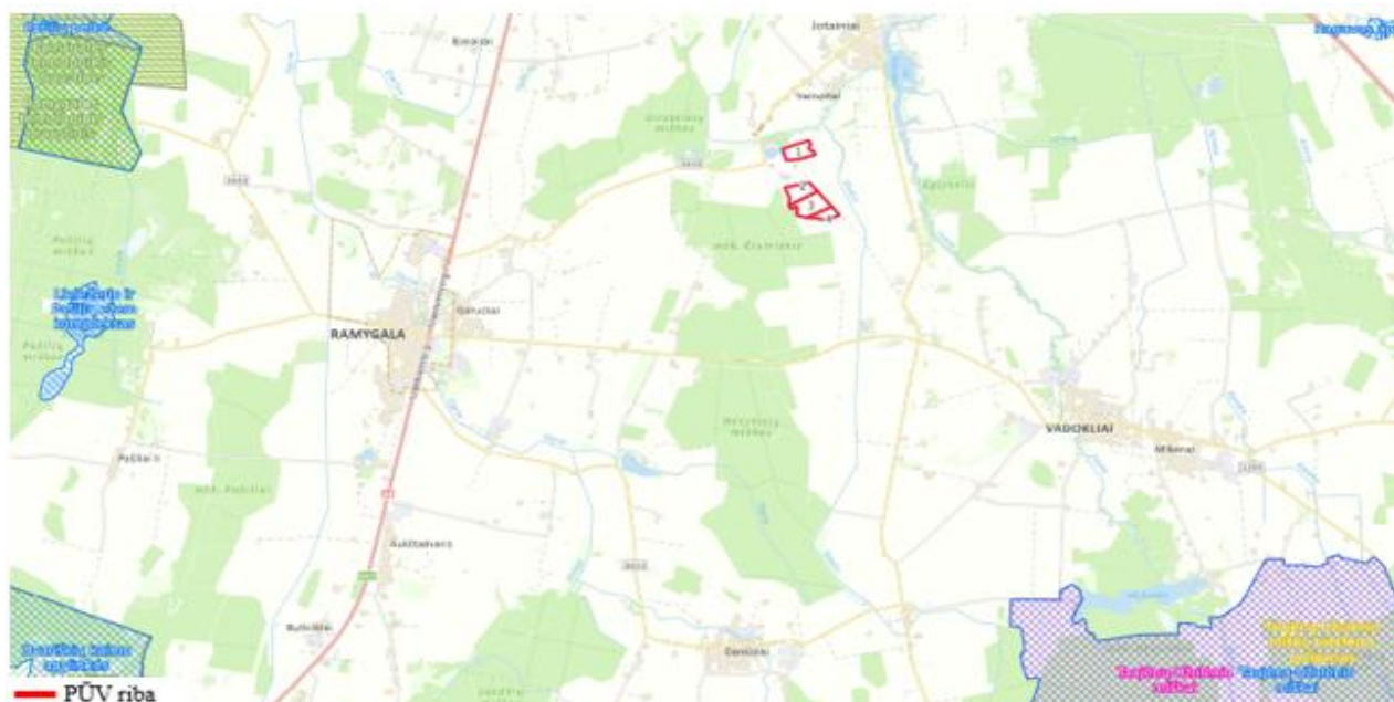
2.20 pav. Ištrauka iš Saugomų teritorijų valstybės kadastro žemėlapis (Šaltinis: https://stvk.lt/map/ )
