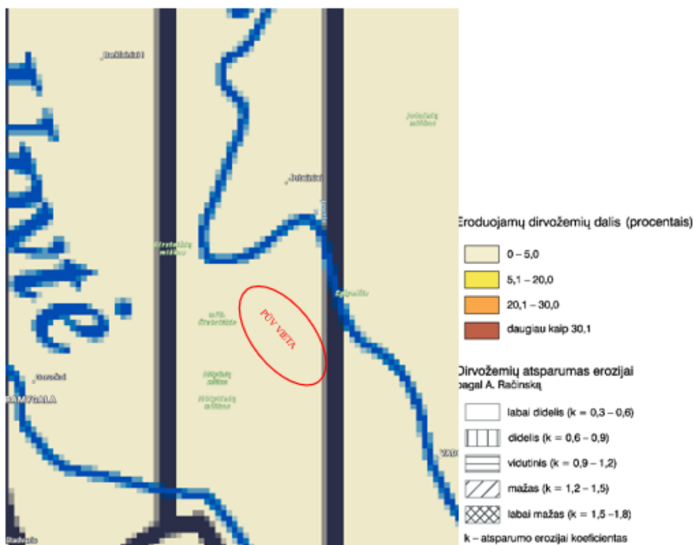
2.7 pav. Ištrauka iš erozijos intensyvumo žemėlapiu
