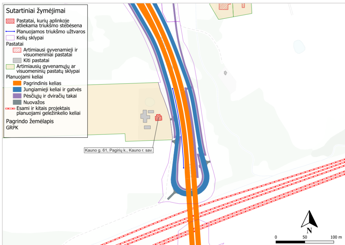
2 pav. Planuojamo kelio 12+960 km esantis pastatas, kurio aplinkoje atliekama triukšmo stebėsena
