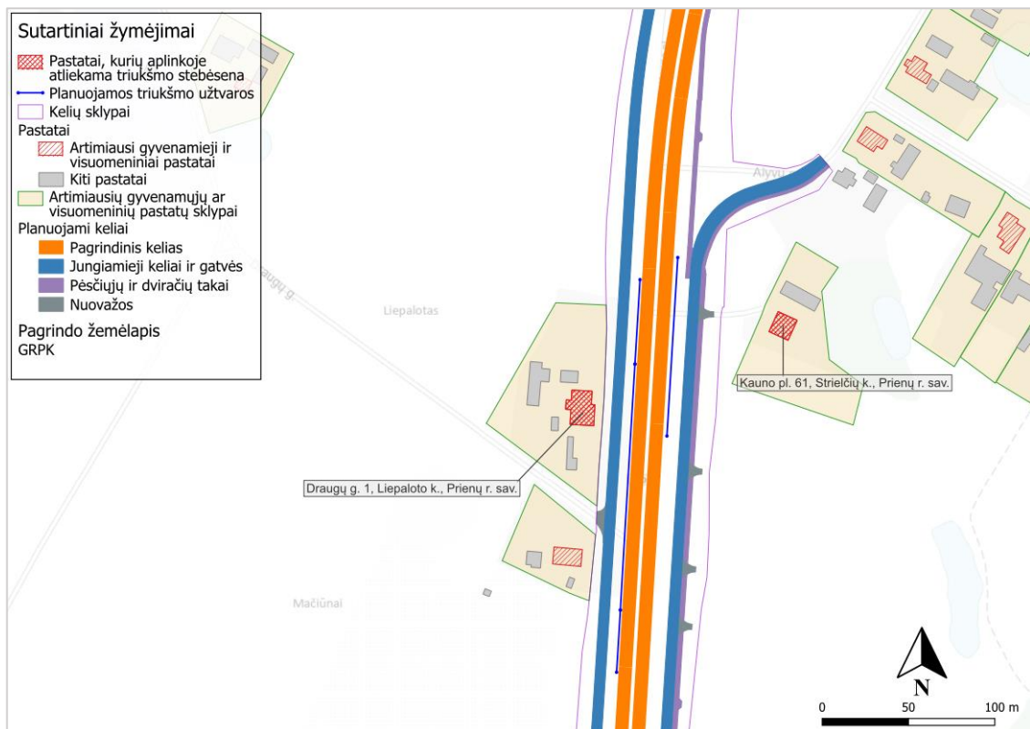
18 pav. Planuojamo kelio 29+500–29+540 km esantys pastatai, kurių aplinkoje atliekama triukšmo stebėsena
