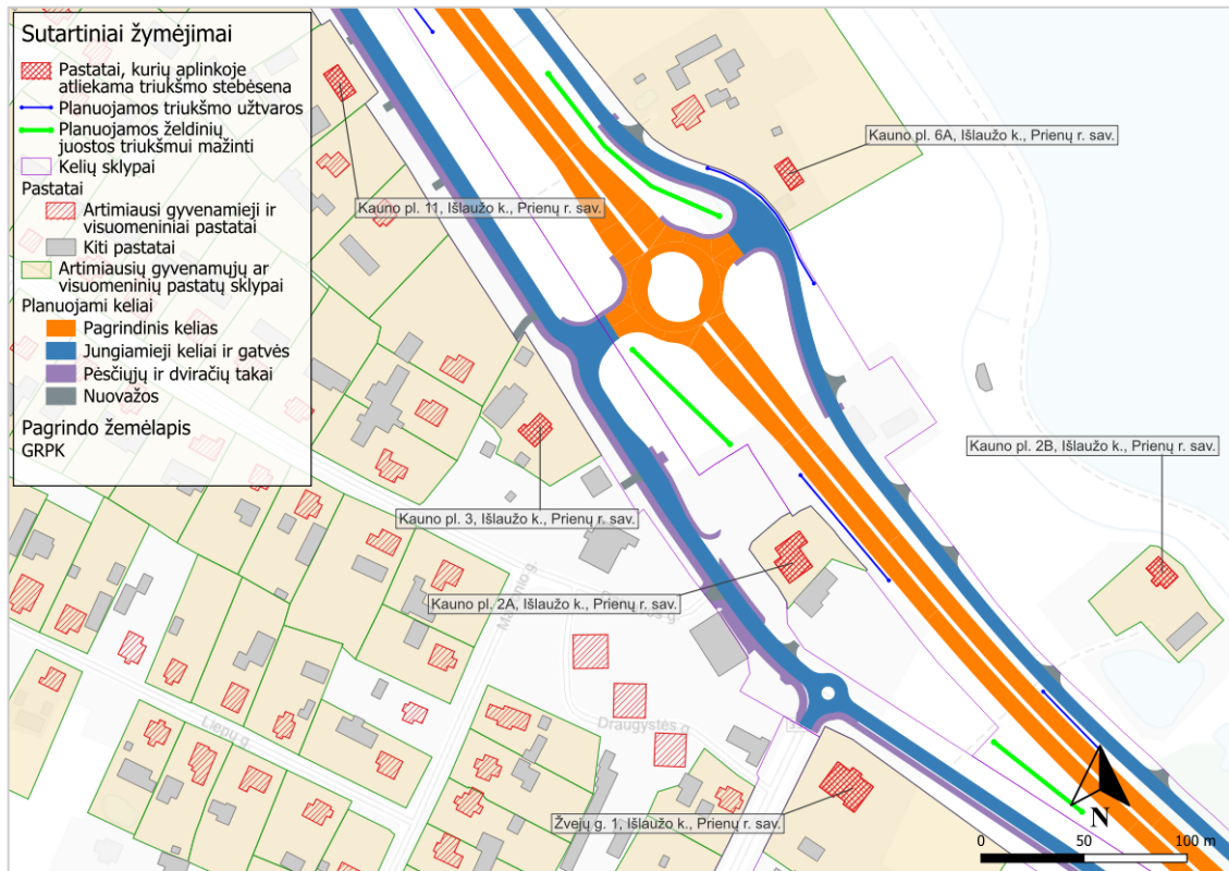
9 pav. Planuojamo kelio 20+440–20+880 km esantys pastatai, kurių aplinkoje atliekama triukšmo stebėsena
