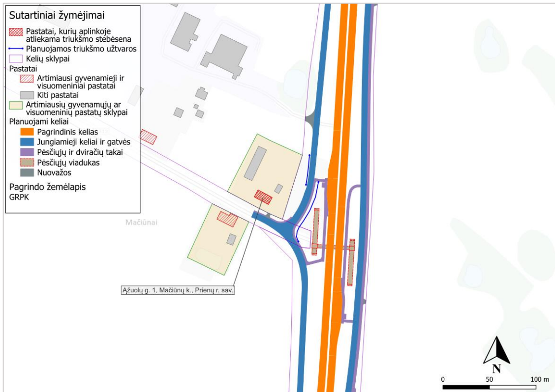
19 pav. Planuojamo kelio 30+100 km esantis pastatas, kurio aplinkoje atliekama triukšmo stebėseną
