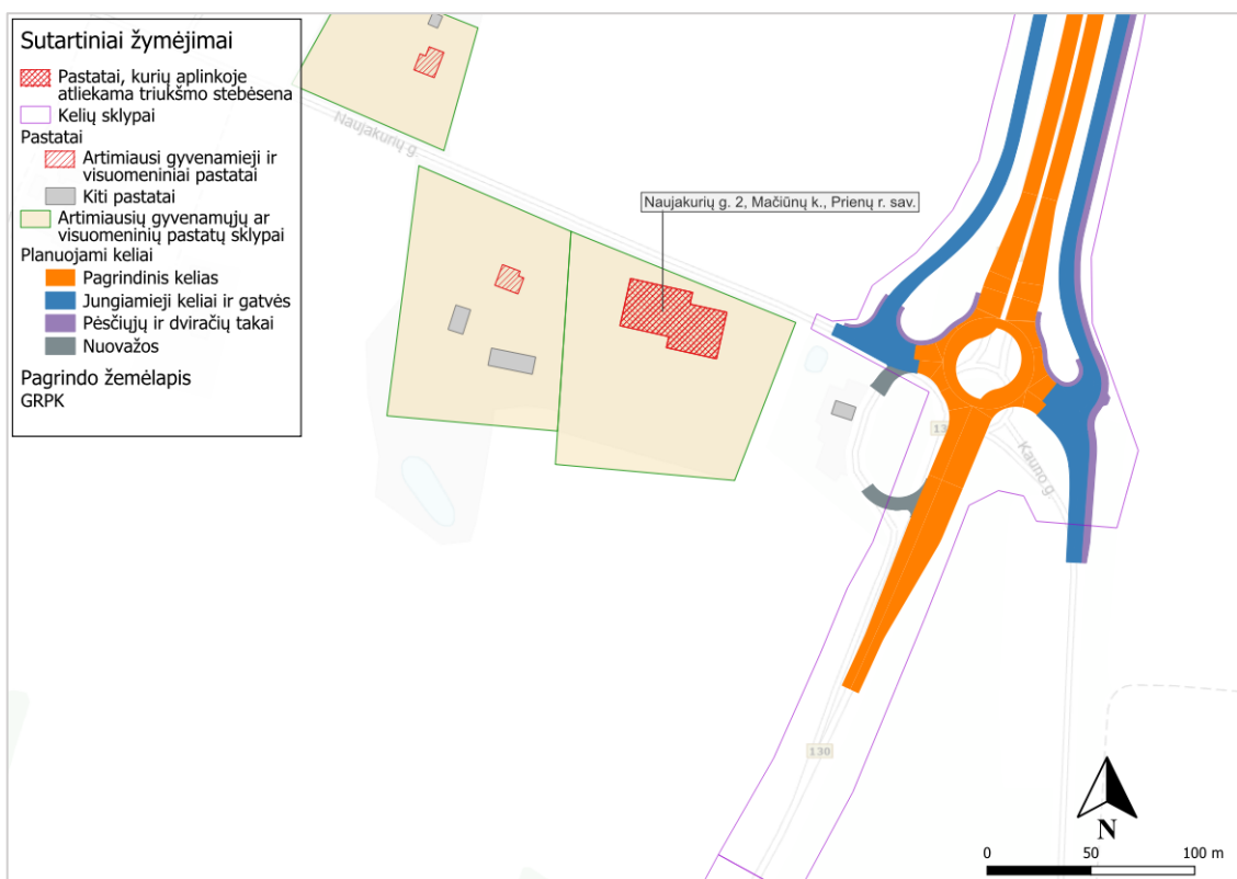
20 pav. Planuojamo kelio 30+680 km esantis pastatas, kurio aplinkoje atliekama triukšmo stebėseną
