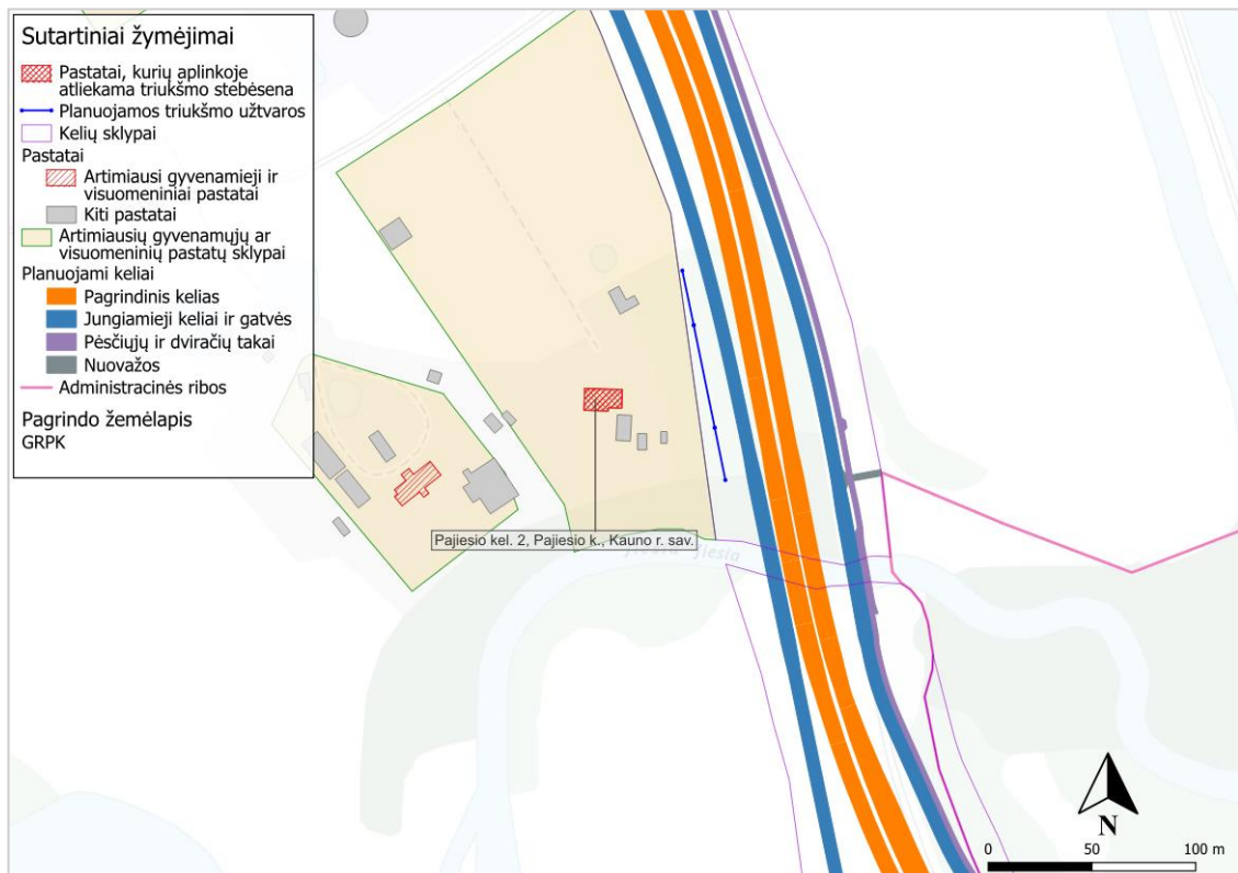
8 pav. Planuojamo kelio 18+800 km esantis pastatas, kurio aplinkoje atliekama triukšmo stebėseną
