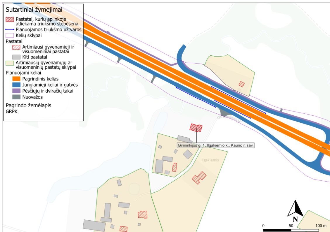
6 pav. Planuojamo kelio 16+600 km esantis pastatas, kurio aplinkoje atliekama triukšmo stebėseną
