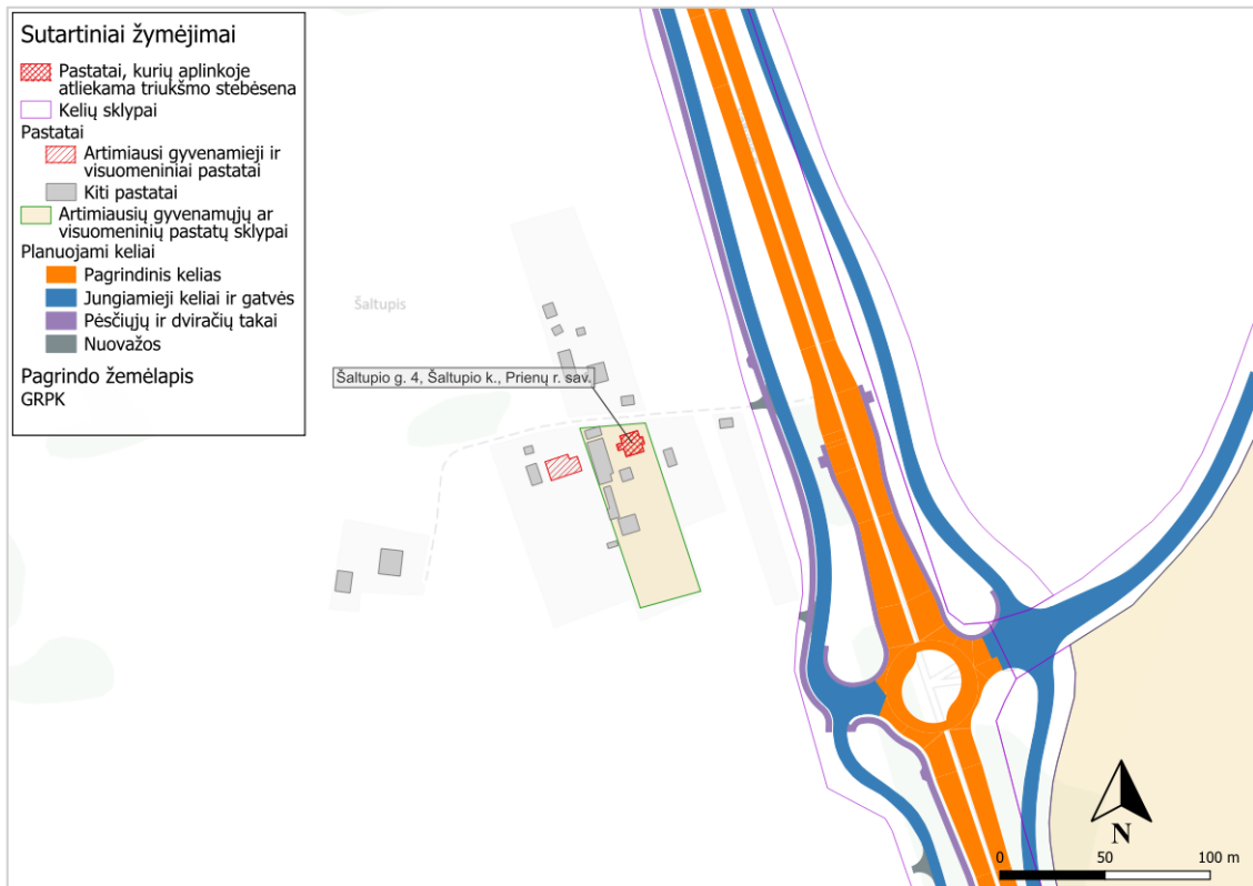
11 pav. Planuojamo kelio 23+200 km esantis pastatas, kurio aplinkoje atliekama triukšmo stebėseną
