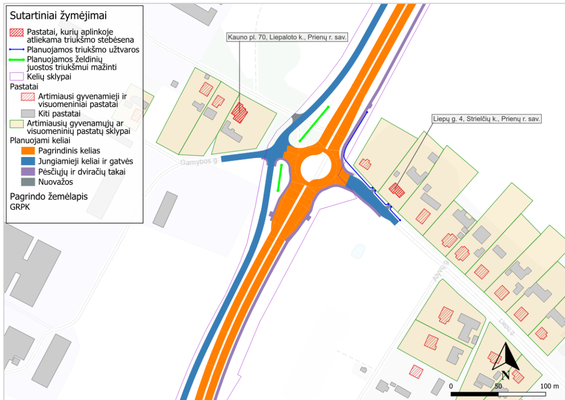
17 pav. Planuojamo kelio 28+920 km esantys pastatai, kurių aplinkoje atliekama triukšmo stebėsena
