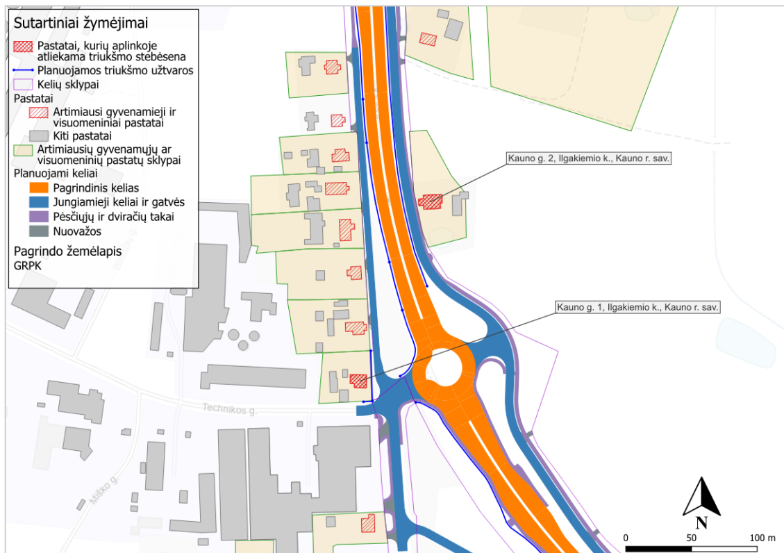
4 pav. Planuojamo kelio 15+200–15+300 km esantys pastatai, kurių aplinkoje atliekama triukšmo stebėsena
