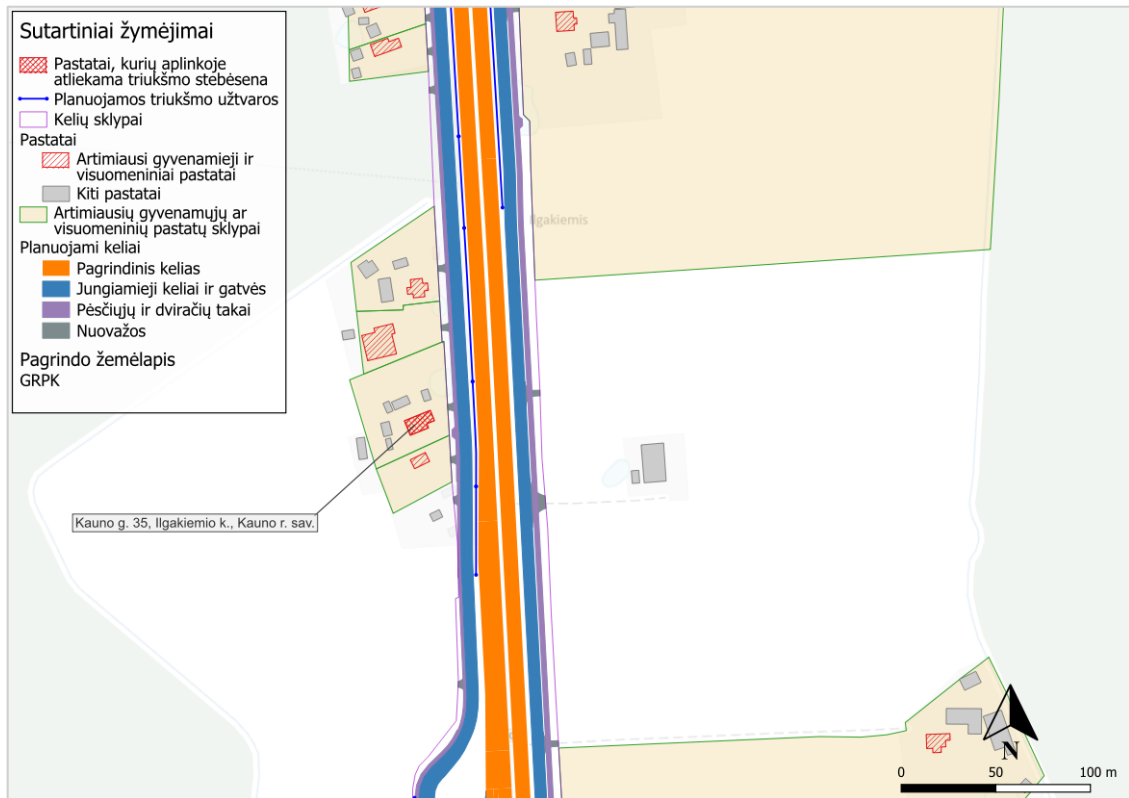
3 pav. Planuojamo kelio 14+380 km esantis pastatas, kurio aplinkoje atliekama triukšmo stebėsena
