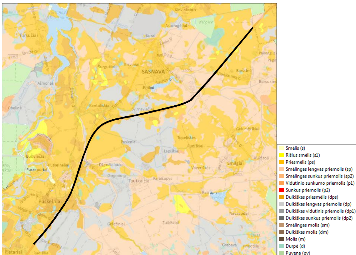
5 pav. Paviršiaus granulimetrinė sudėtis pagal Fere rekonstruojamo kelio (pažymėta juodai) aplinkoje (šaltinis: https://www.geoportal.lt ).
