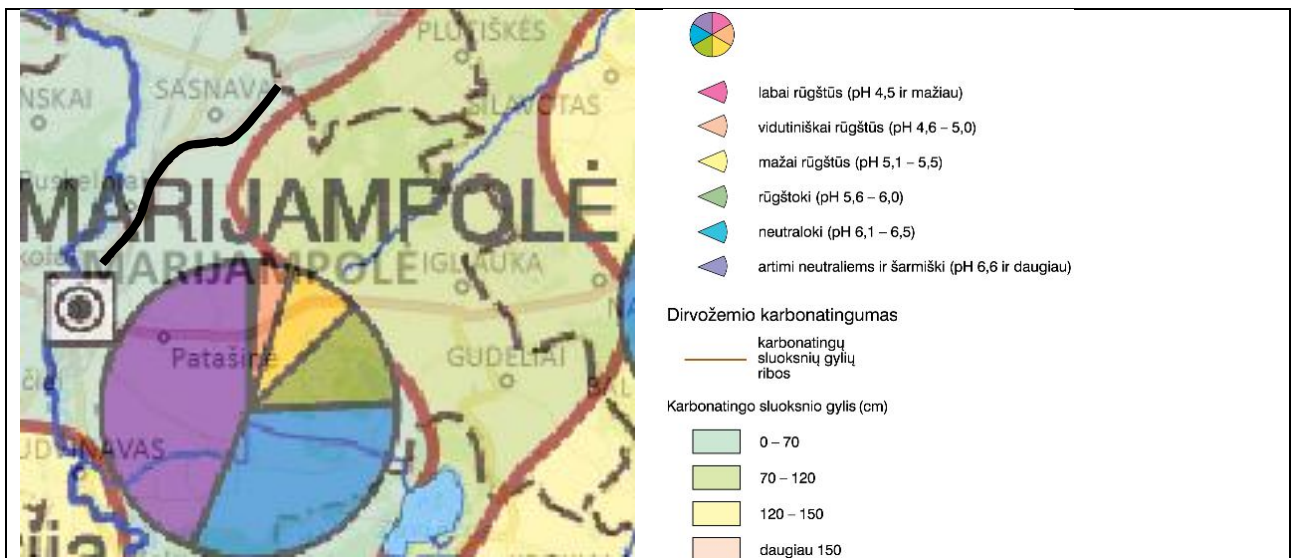
2 pav. Dirvožemio karbonatingumas ir rūgštingumas rekonstruojamo kelio (pažymėta juodai) aplinkoje (šaltinis: https://www.geoportal.lt ).
