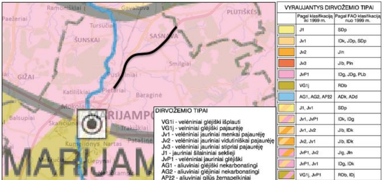
1 pav. Vyraujantys dirvožemio tipai rekonstruojamo kelio (pažymėta juodai) aplinkoje (šaltinis: https://www.geoportal.lt ).
