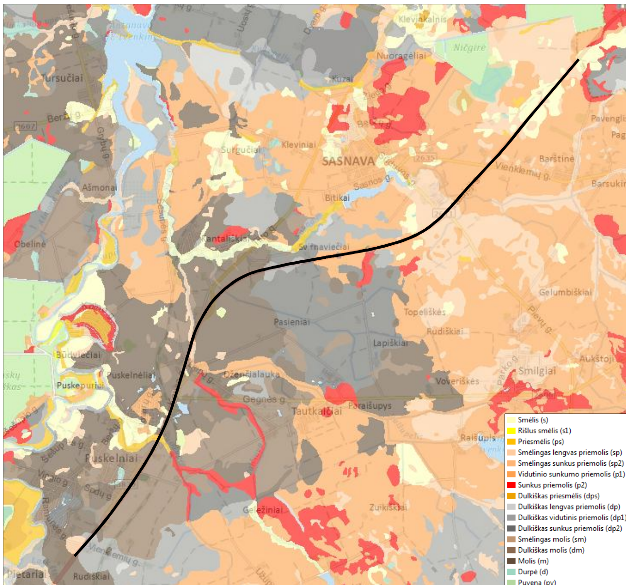
6 pav. Vyraujanti dirvodarinė granuliometrinė sudėtis pagal Fere rekonstruojamo kelio (pažymėta juodai) aplinkoje (šaltinis: https://www.geoportal.lt ).
