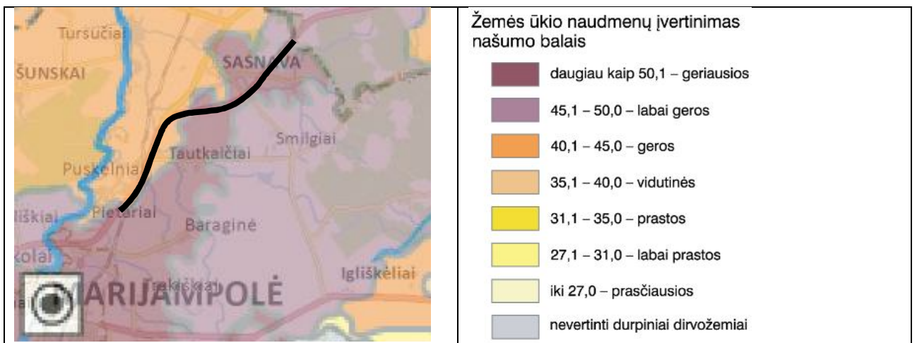
3 pav. Dirvožemio bonitavimas rekonstruojamo kelio (pažymėta juodai) aplinkoje (šaltinis: https://www.geoportal.lt ).
