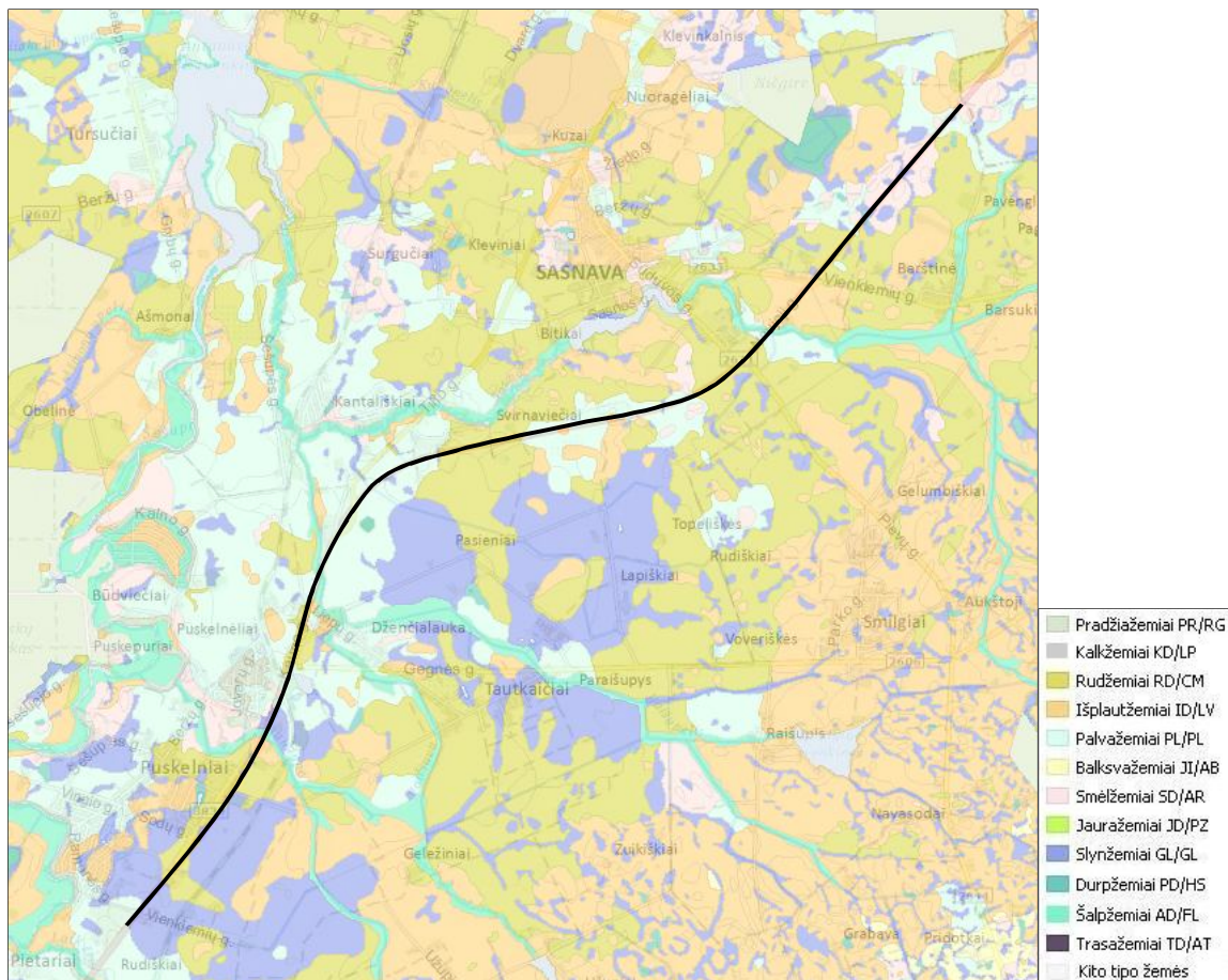
4 pav. Dirvožemio tipai rekonstruojamo kelio (pažymėta juodai) aplinkoje (šaltinis: https://www.geoportal.lt ).
